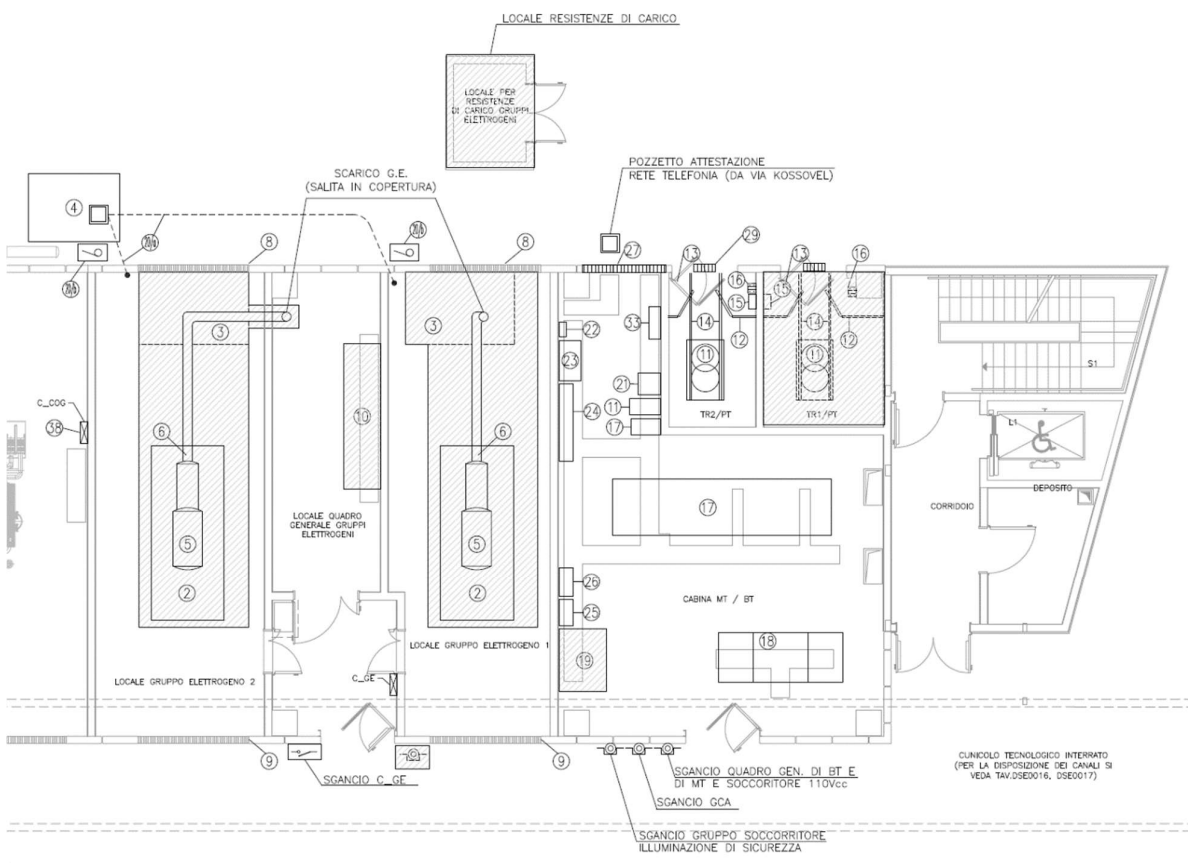
Figura 6. Estratto della planimetria della centrale tecnologica di Basovizza.
