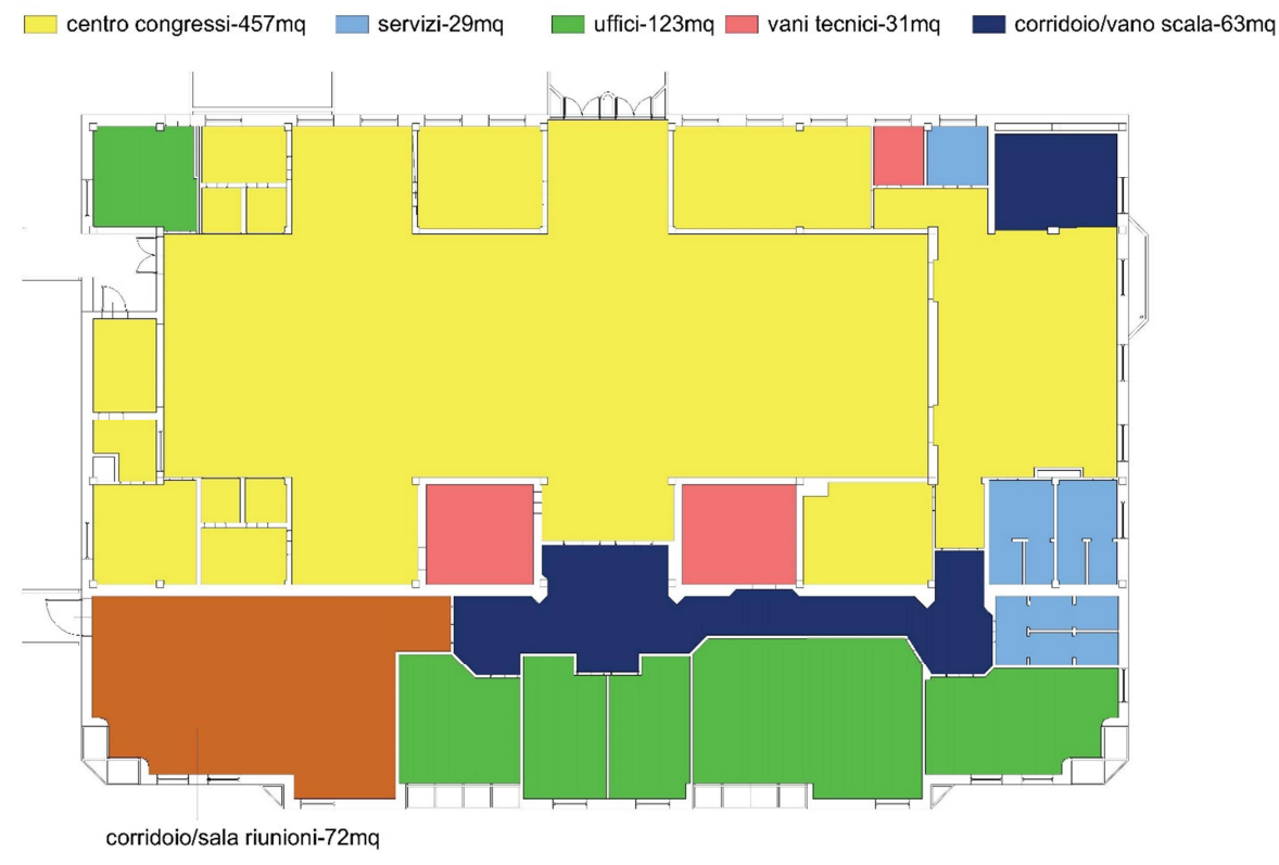
Figura 19. Superfici e destinazioni d'uso previsto nel progetto di riqualificazione del centro congressi.
