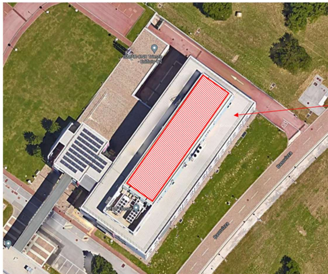
Figura 14. Collocazione dell'impianto sulla copertura dell'edificio "Q2".
